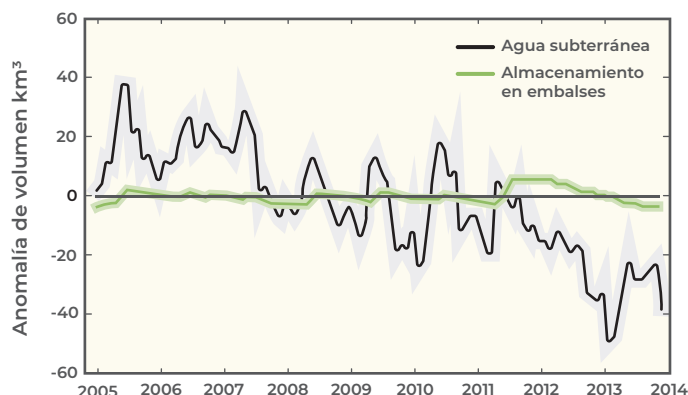
FIGURA 2. Anomalías mensuales de almacenamiento de aguas subterráneas (negro) y de almacenamiento superficial (verde), para toda la cuenca del río Colorado de diciembre de 2004 a noviembre de 2013.
